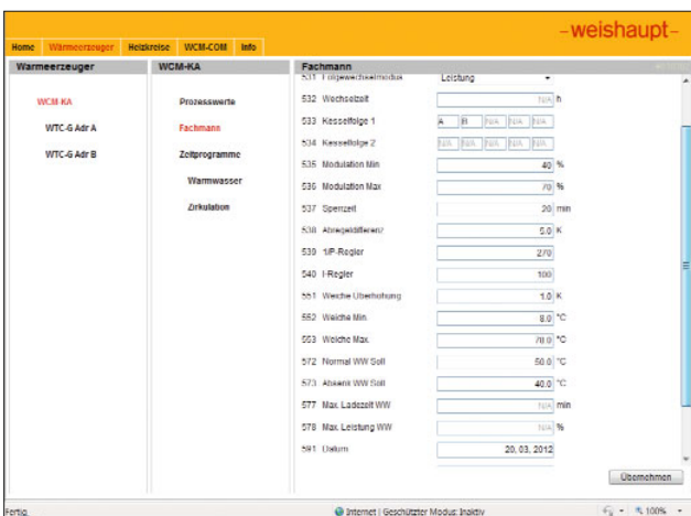
Änderungen von Anlagenparametern erfolgen über die zweite Bedienebene
